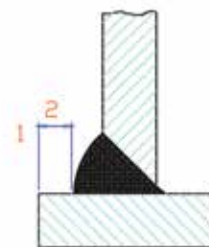
B. Kaynak Sonrası
