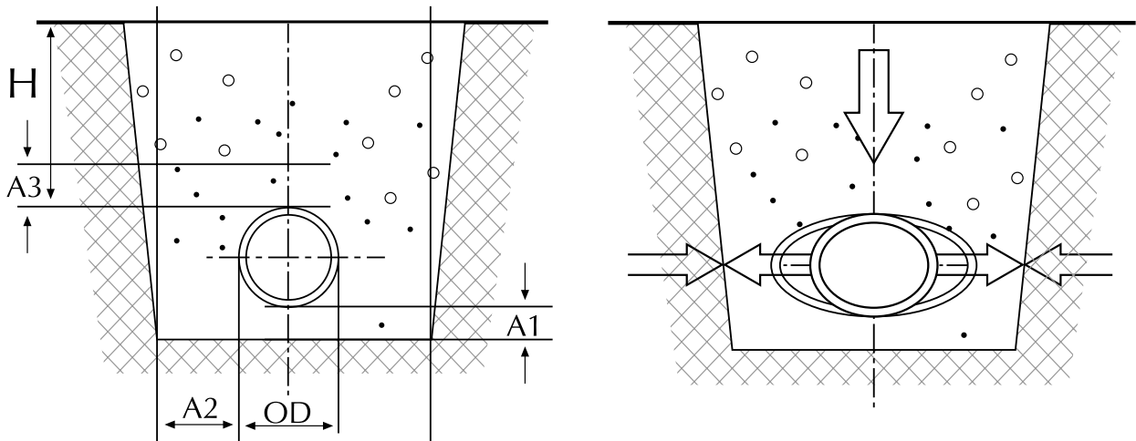
Kanal İçinde Borunun Yerleşimi
