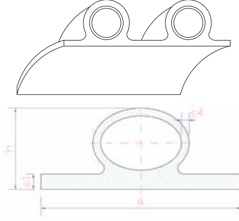
PR serisi FKS borularının cidar kesiti ve teknik yapısı
