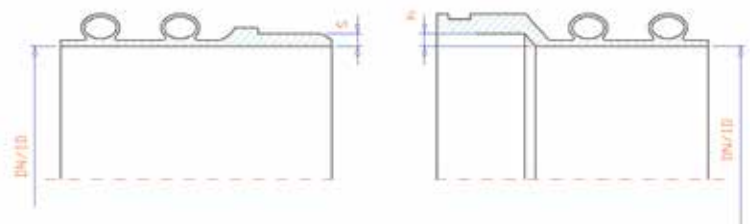
FKS boru elektrofüzyon kaynak birleşim nokta kesidi.
