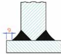
B. Kaynak Sonrası
