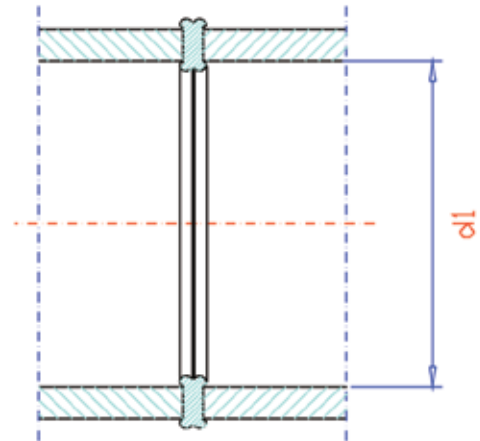
FKS boru alın kaynak birleşim nokta kesidi.
