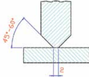
A. Kaynak Öncesi
